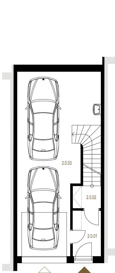
1. NADZEMNÍ PODLAŽÍ
