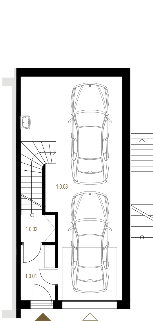
1. NADZEMNÍ PODLAŽÍ
