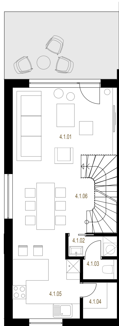
2. NADZEMNÍ PODLAŽÍ
